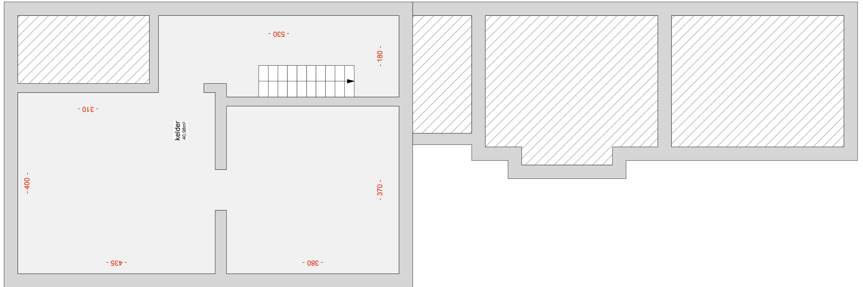
GRONDPLAN kelder
