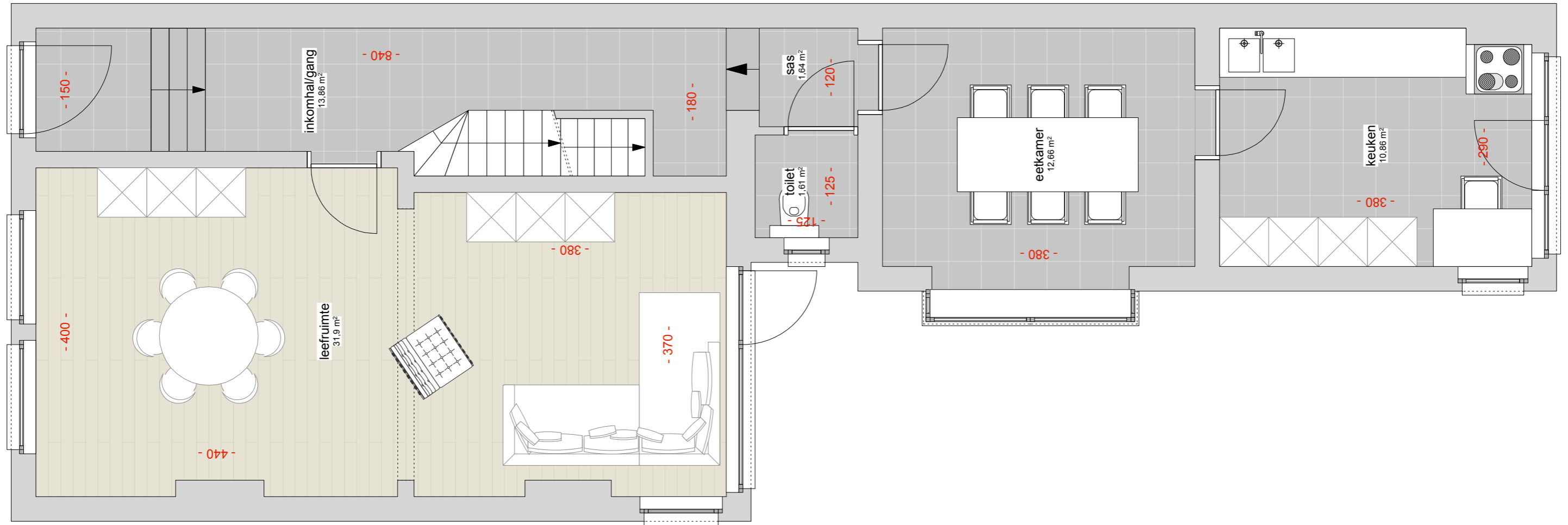
GRONDPLAN gelijkvloers
