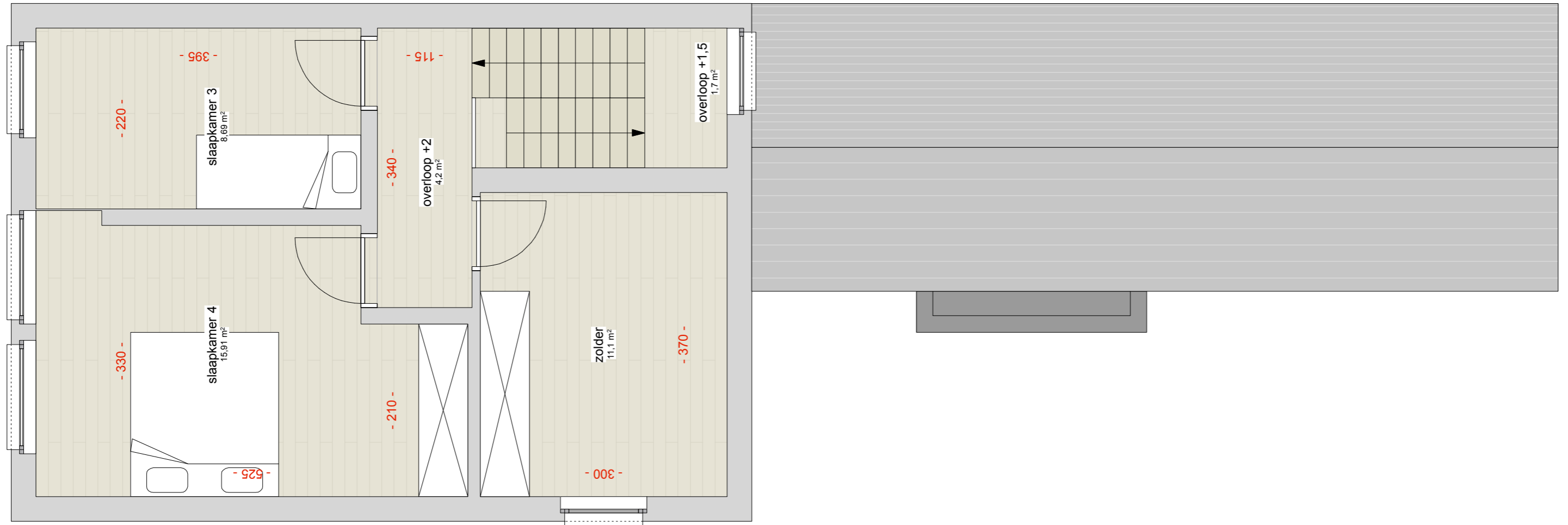
GRONDPLAN verdieping 2
